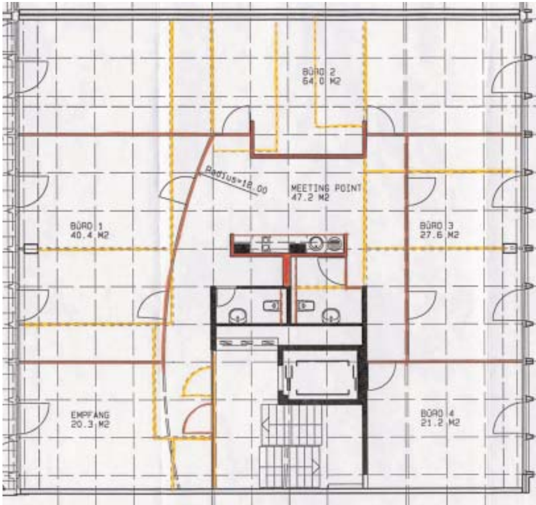
Grundriss 2. Obergeschoss
